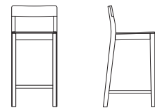
Wooden seat // Holzsitz Frame // Gestell h 65
